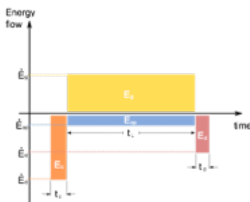
Figura 1. Flujos energéticos
